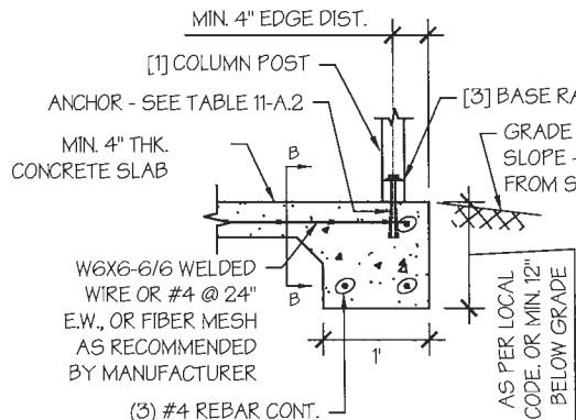
STANDARD EDGE DETAIL
